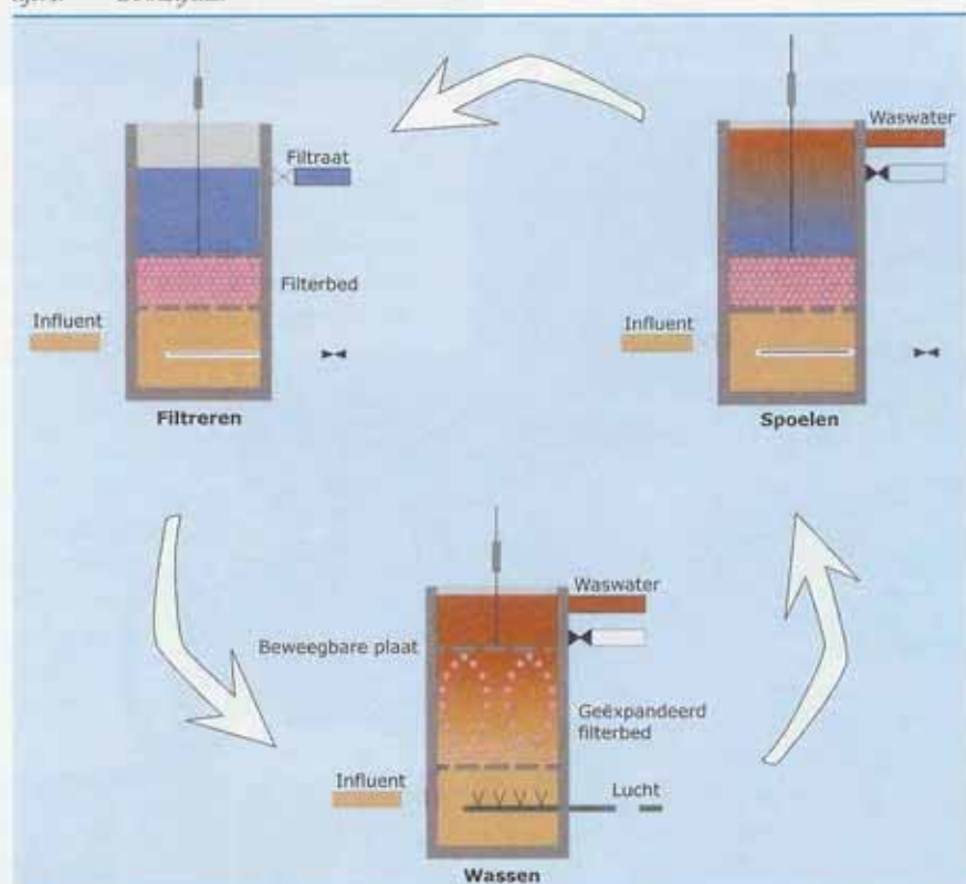
Afb. 1: De wascyclus.
